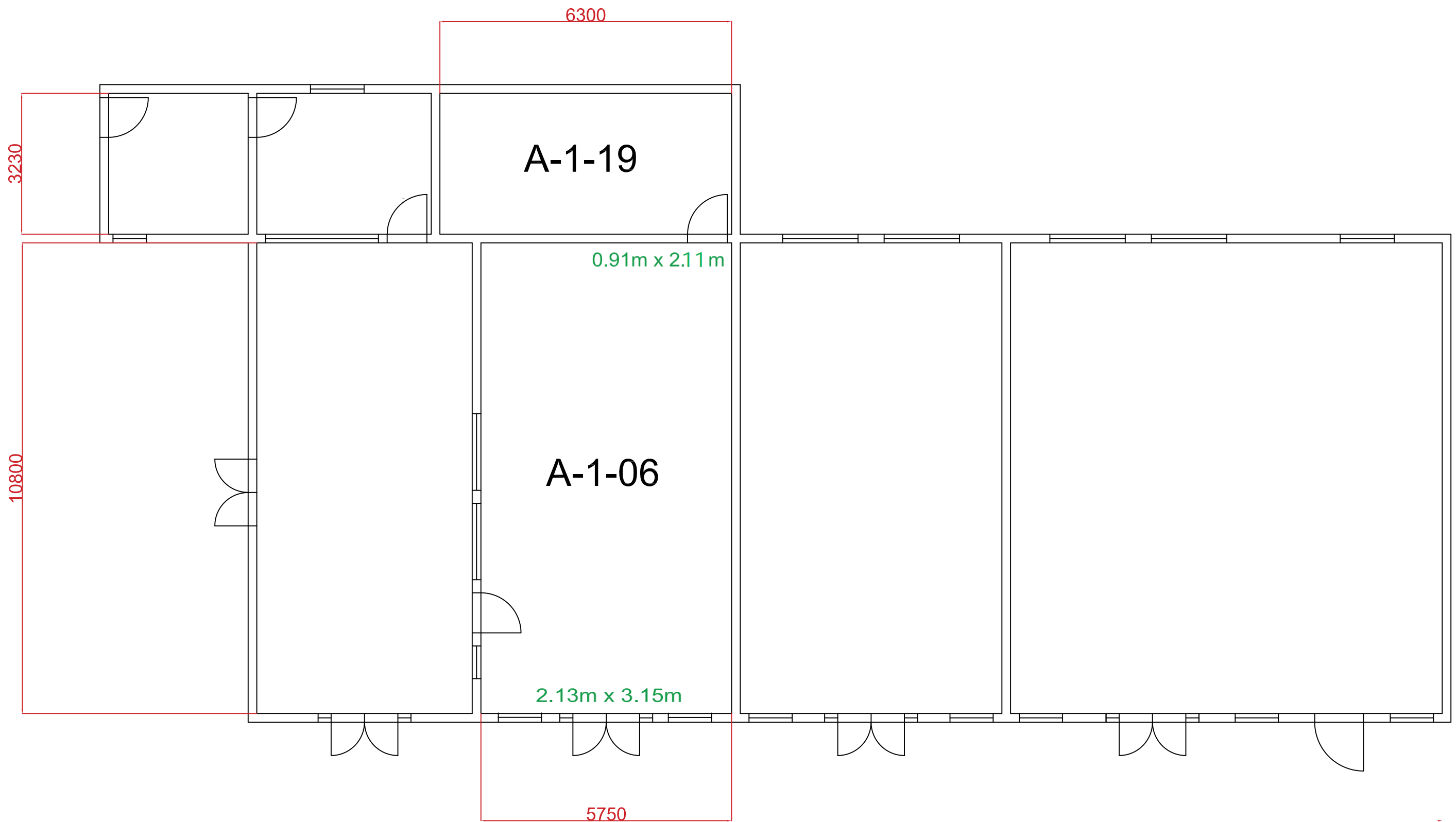
房間、門尺寸圖
